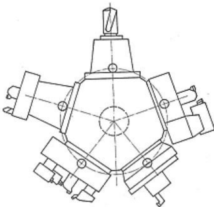
Obr. 2: Nákres revolverové hlavy
