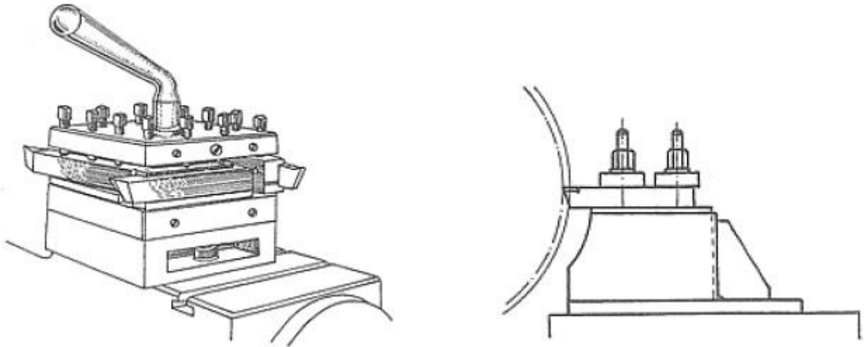
Obr. 1: Upnutí nože na otočnou nožovou hlavu (vlevo), upnutí na upínky (vpravo).
